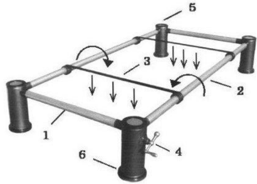
Рис. 2. Принцип роботи спускового механізму
