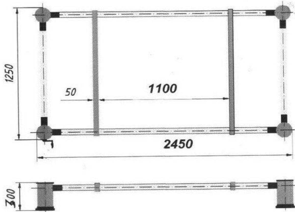
Рис. 1. Креслення спускового механізму
